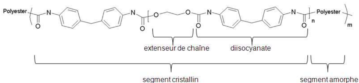
Figure 14 : Molécule de polyuréthane segmenté
