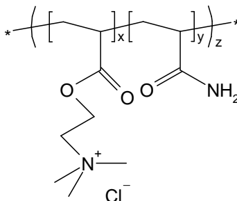
Figure 5 : Copolymère cationique
