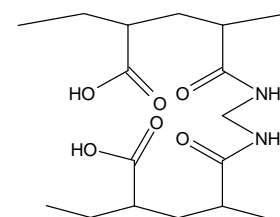
Figure 3 : Copolymère réticulé
