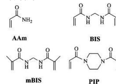
Figure 3 : Copolymère réticulé
