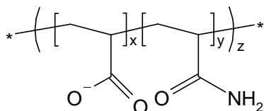
Figure 4 : Copolymère anionique
