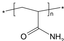
Figure 1 : Polyacrylamide non-ionique
