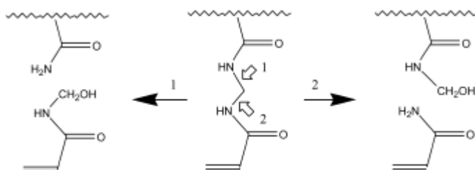
Figure 16 : Deux voies d'hydrolyse possibles pour le méthylène bisacrylamide dont une des deux insaturations seulement intègre la chaîne [10]
